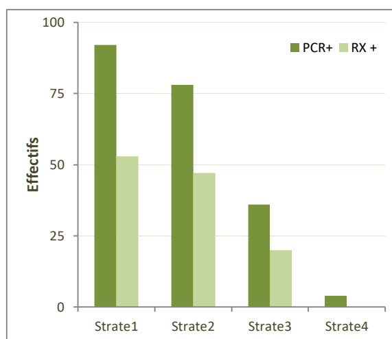
Graph 9 : Répartition des patients traités selon la méthode diagnostique au 27 avril
