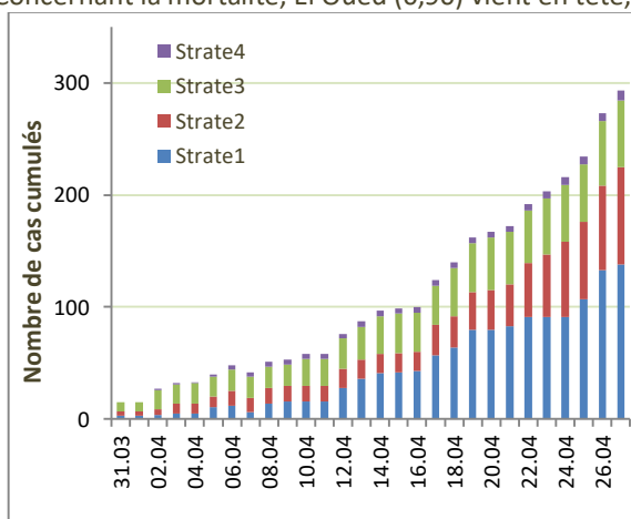
Graph 3 : Evolution des cas cumulés par strates de la région Sud 27 avril 2020
