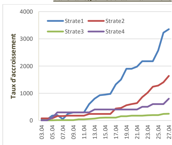
Graph 5 : Evolution des taux d'accroissement dans la région Sud au 27 avril 2020
