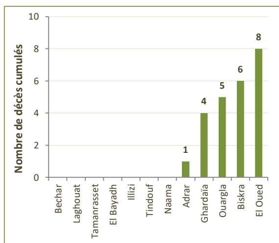
Graphe 7 : Répartition des décès cumulés des wilayas de la région Sud au 27 avril
