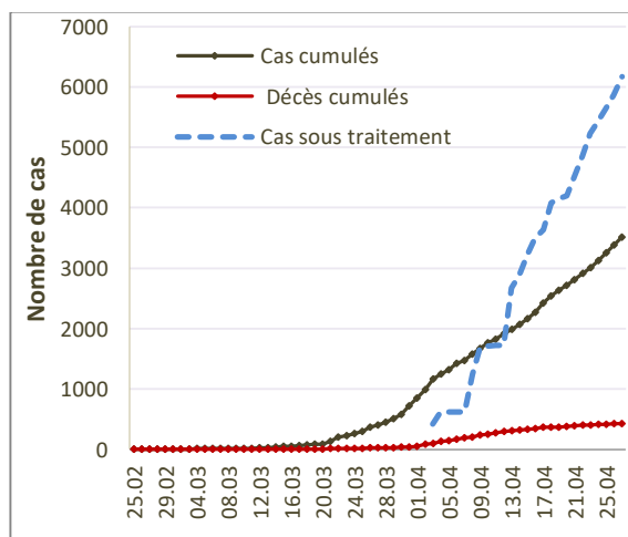
Graph 2 : Evolution des cas et décès cumulés, et des patients sous traitement au 27 avril
