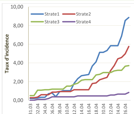
Graph 4 : Evolution des taux d'incidence dans la région Sud au 27 avril 2020
