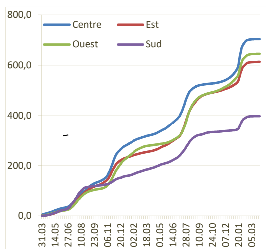
Graph 6 : Evolution du taux d'incidence cumulé par région sanitaire au 01.04
